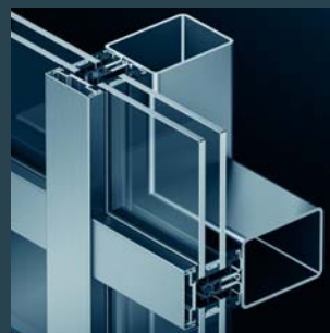
SCHÜCO FW 50+ AOS SCHÜCO FW 50+ AOS
