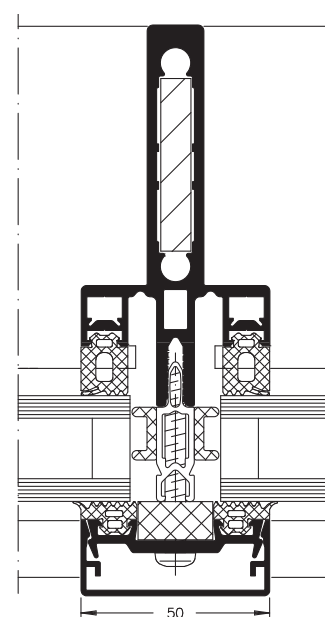
SCHÜCO FW 50+S.HI,
