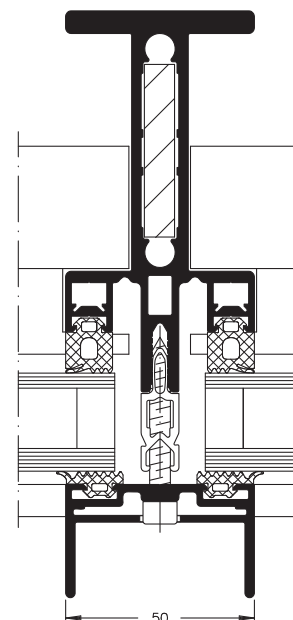
SCHÜCO FW 50+S
