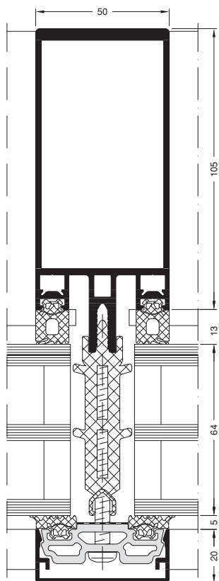
SCHÜCO FW 50+.SI függőnyfal rendszer vízszintes metszete SCHÜCO FW 50+.SI façade system horizontal cut
